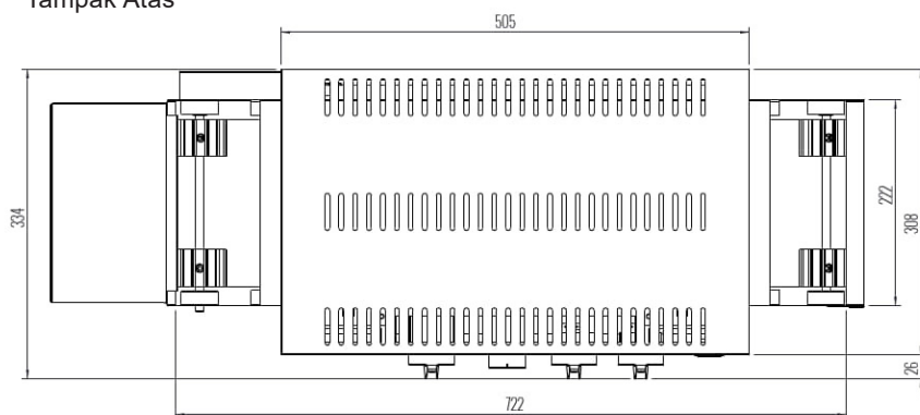
Tampak Atas
