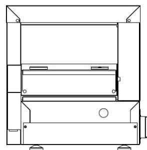
Tampak Belakang
