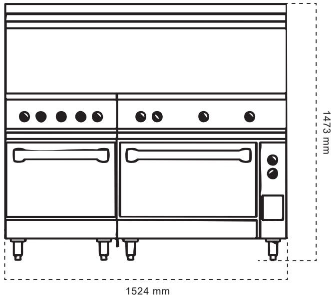
TAMPAK DEPAN
