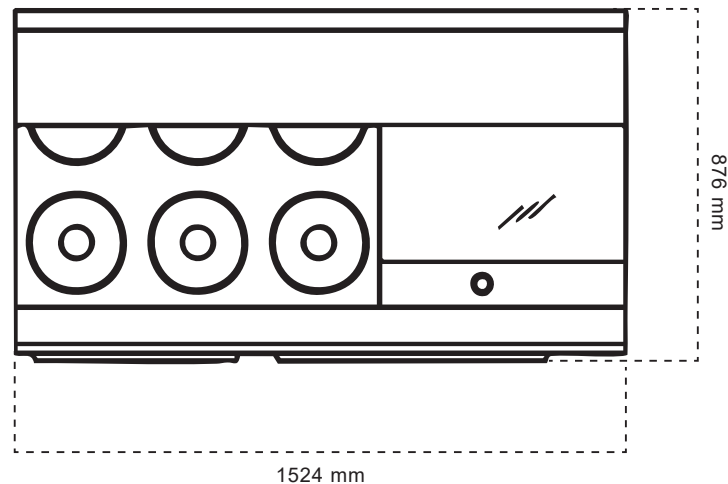
TAMPAK ATAS
