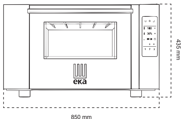
Tampak Depan
