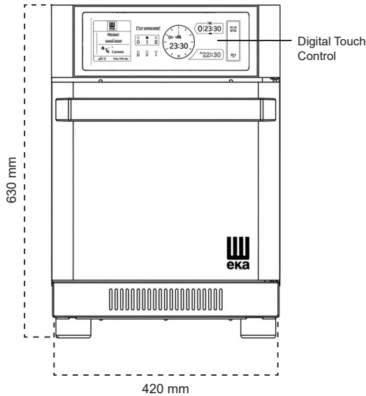
Tampak Depan
