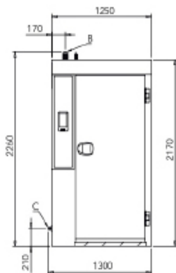
Tampak Depan
