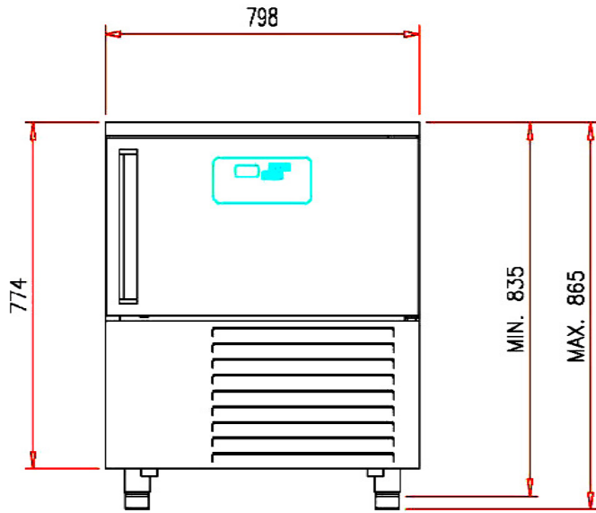
Tampak Depan
