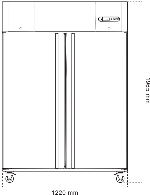
TAMPAK DEPAN
