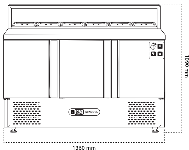
Tampak Depan
