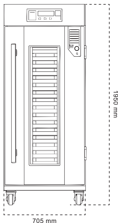
TAMPAK DEPAN
