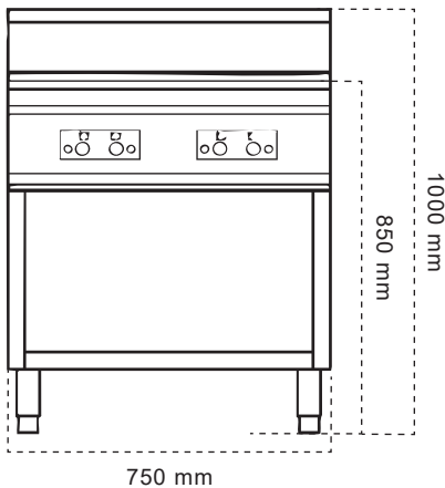
TAMPAK DEPAN
