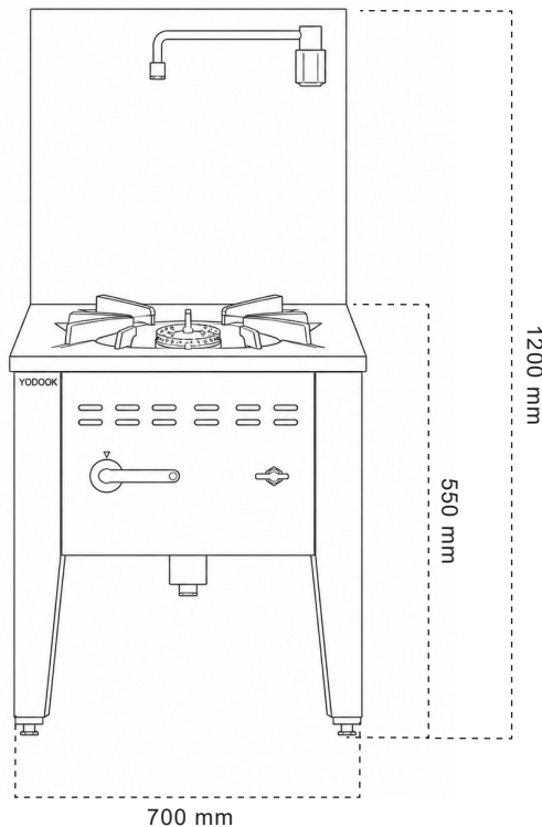
TAMPAK DEPAN
