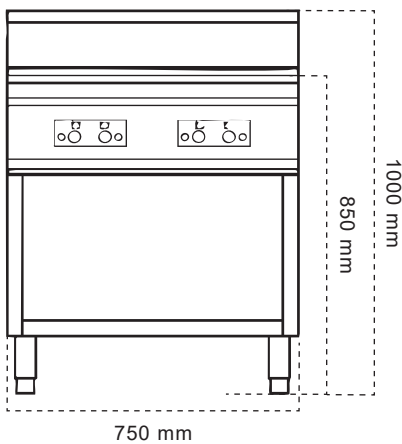
TAMPAK DEPAN
