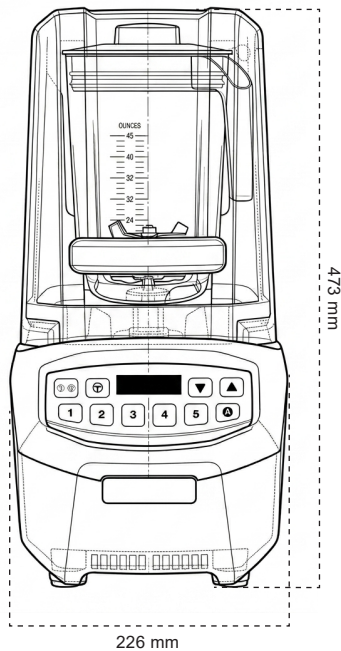
TAMPAK DEPAN
