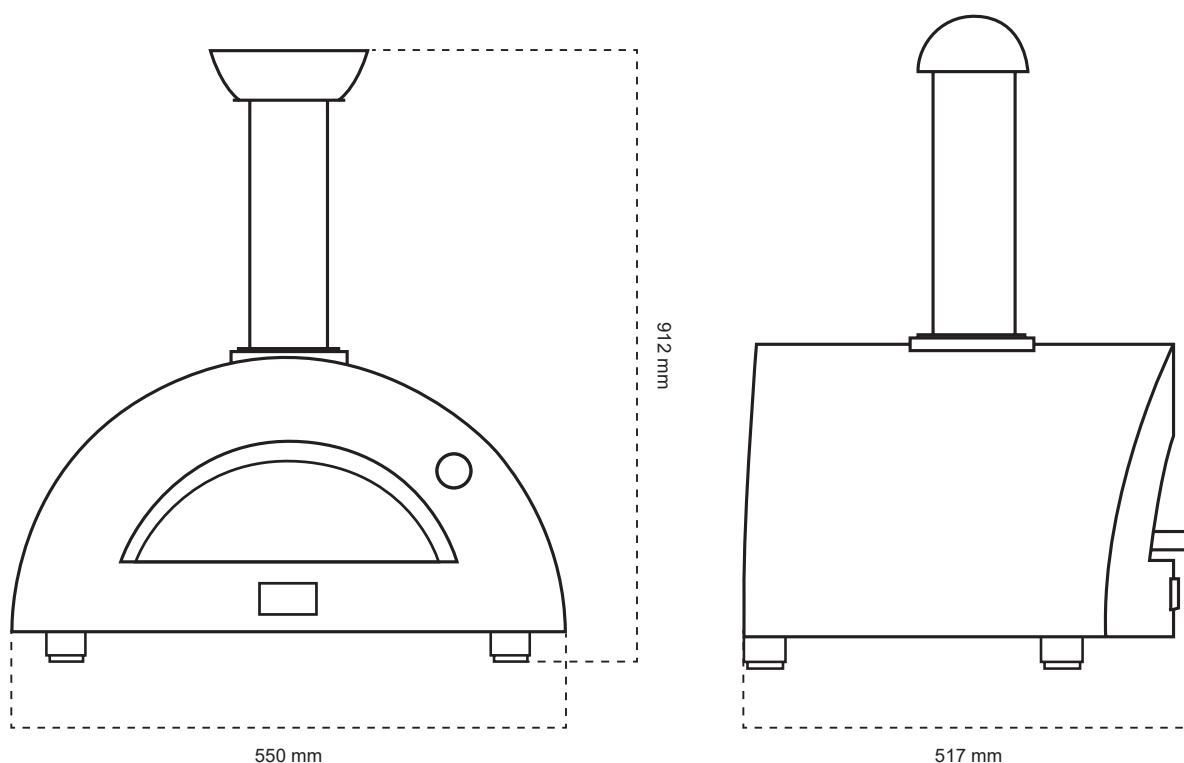
Tampak Depan
