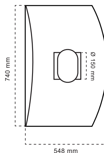
TAMPAK ATAS
