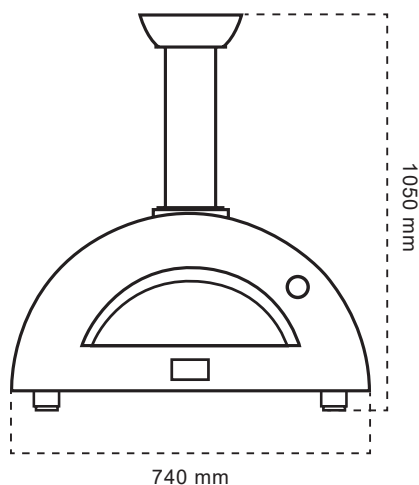
TAMPAK DEPAN
