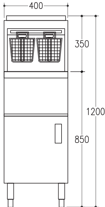
TAMPAK DEPAN
