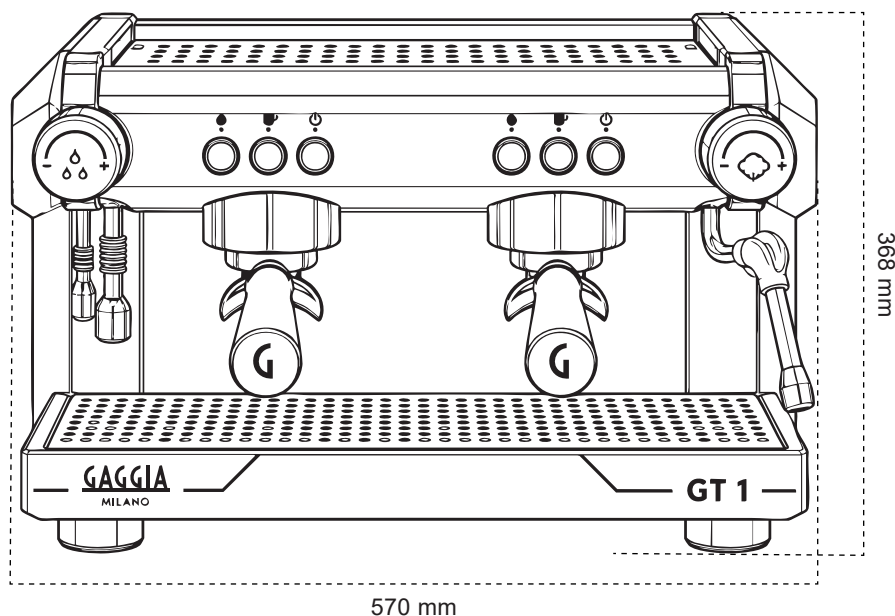
TAMPAK DEPAN
