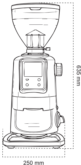
TAMPAK DEPAN
