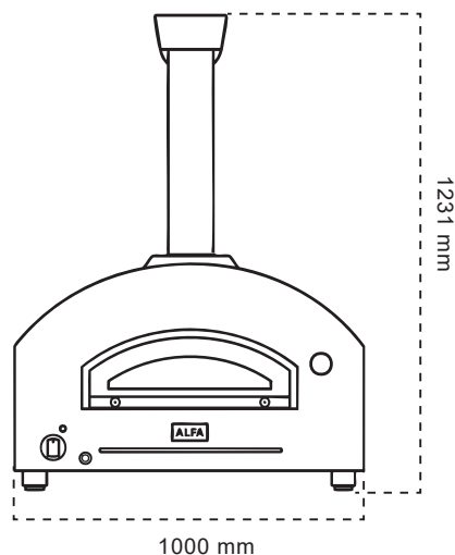
TAMPAK DEPAN
