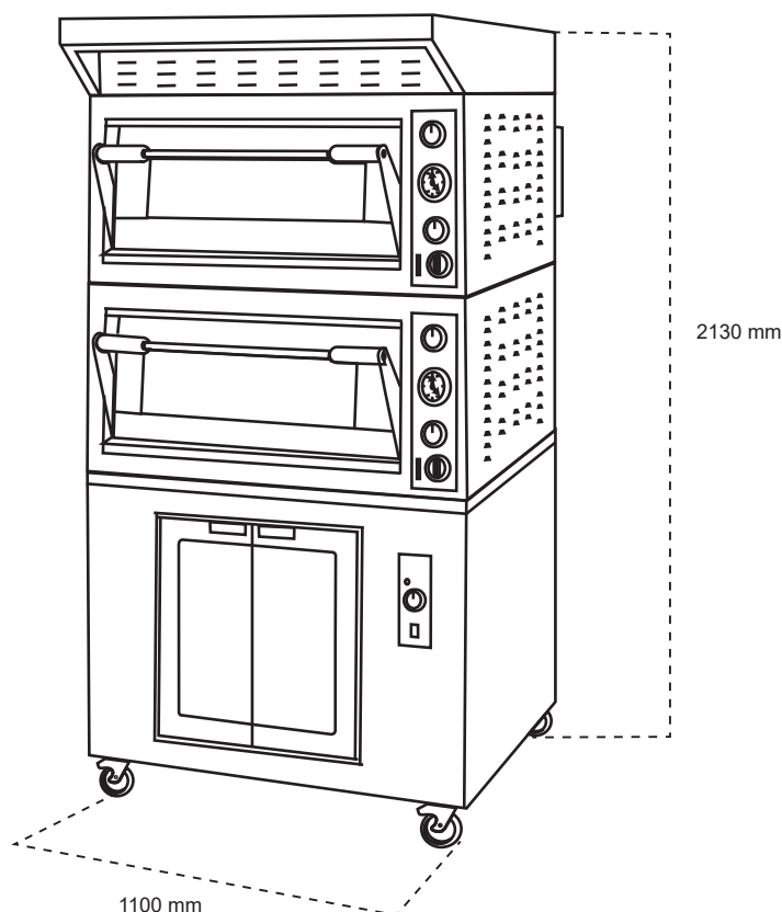
Tampak Depan
