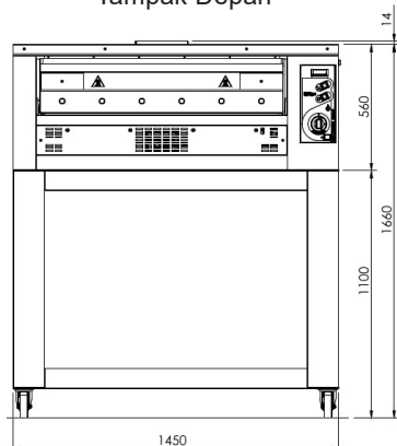
Tampak Depan
