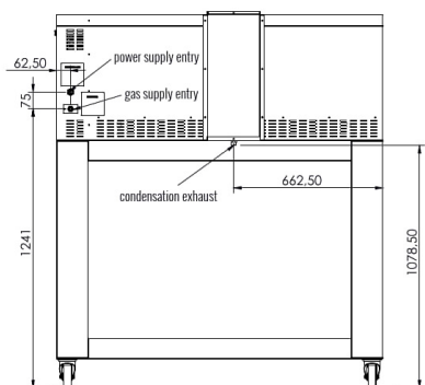
Tampak Belakang
