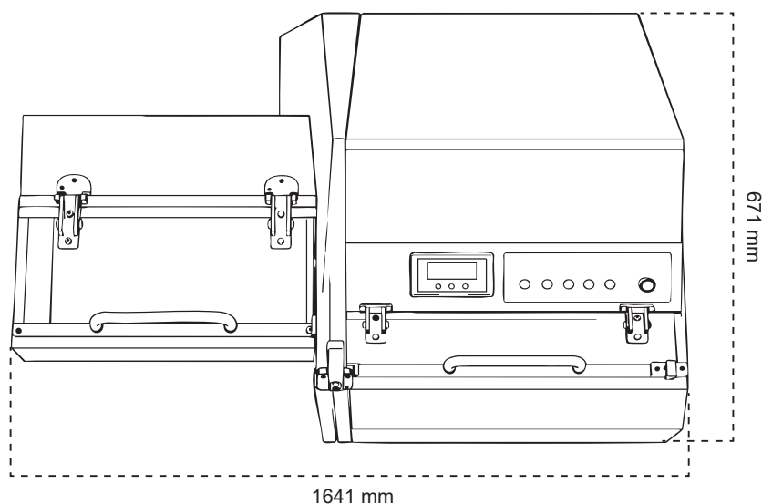
TAMPAK ATAS
