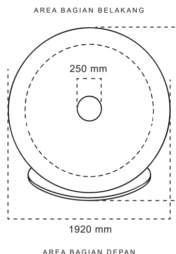
TAMPAK ATAS
