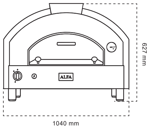
TAMPAK DEPAN
