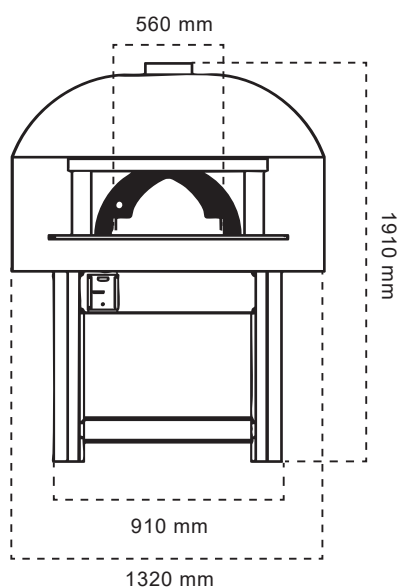
TAMPAK DEPAN
