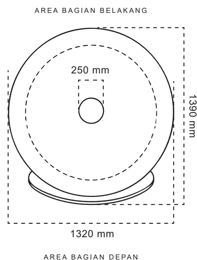
TAMPAK ATAS
