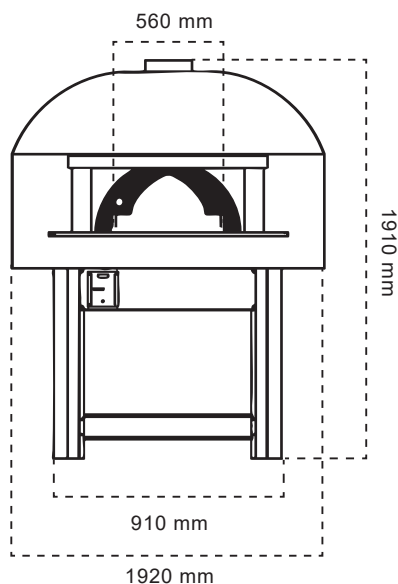
TAMPAK DEPAN
