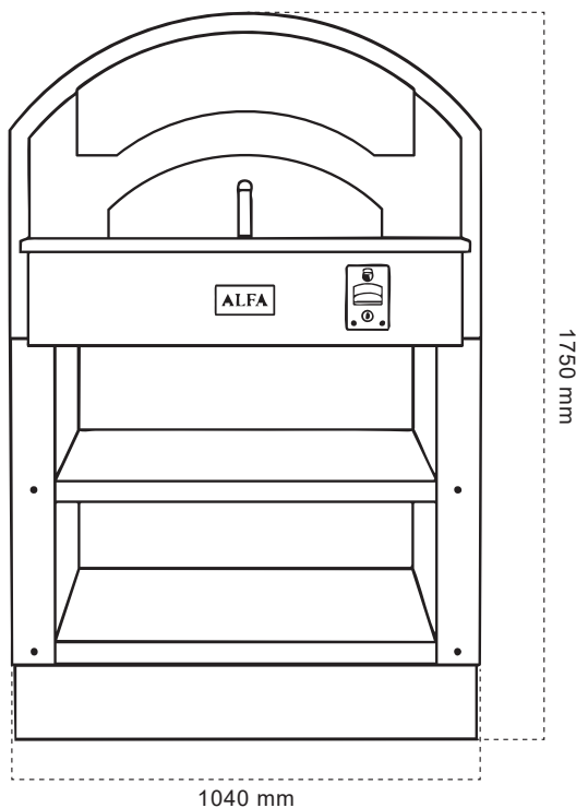
TAMPAK DEPAN
